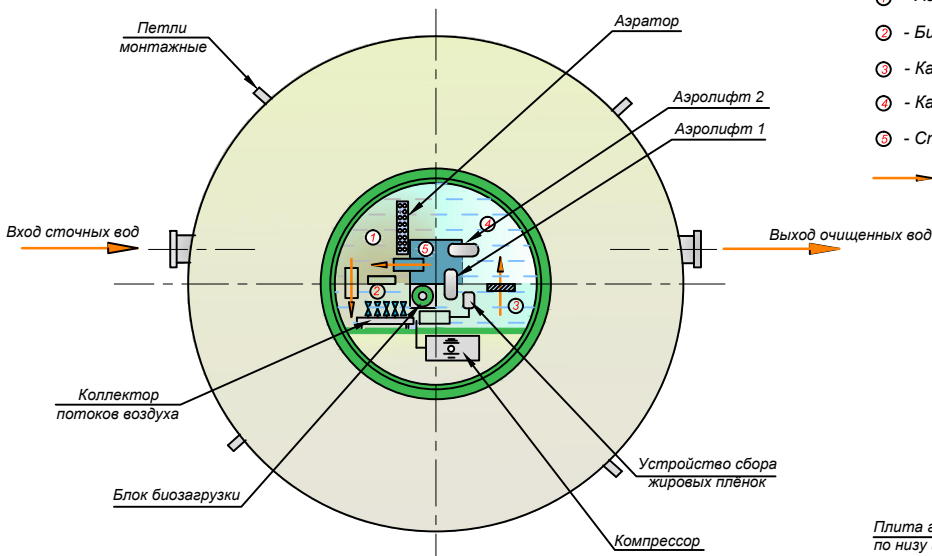
Разрез (без основания) А-А (1:10)
